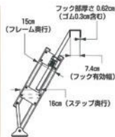
イラストはMTS-40-2-900S
