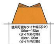
図2 畝上げ機で土上げた状態
